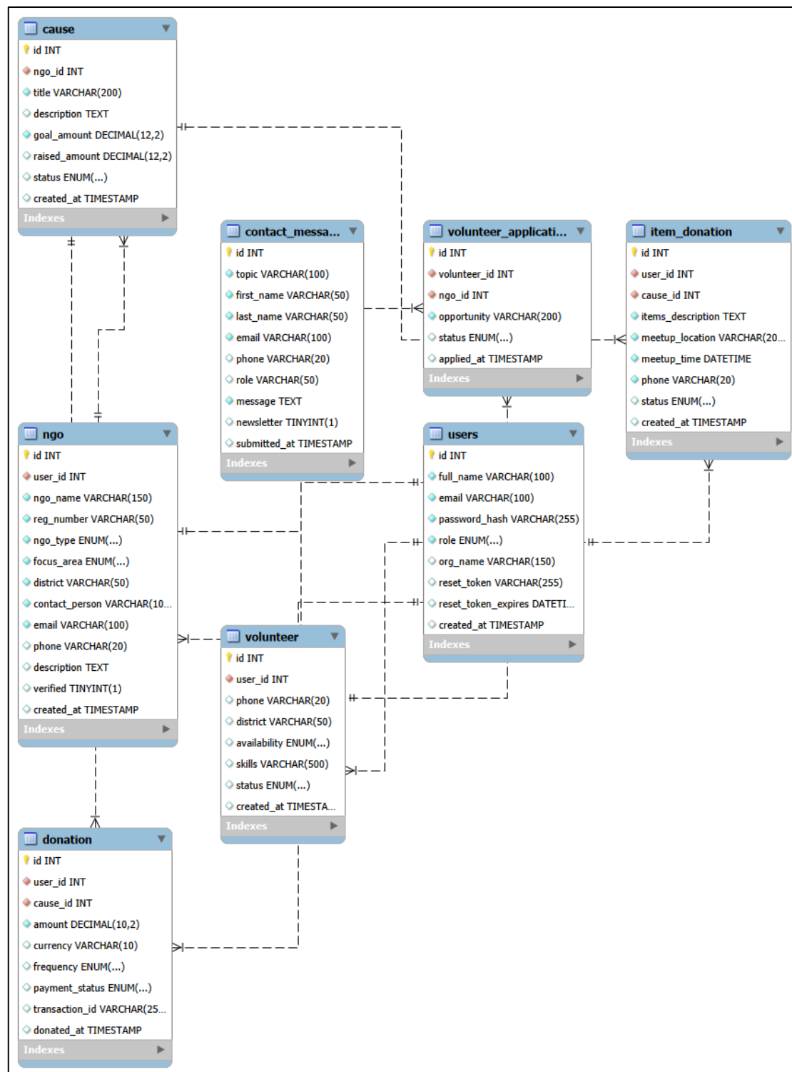
Figure 2: ER Diagram
